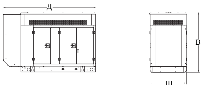
АКУСТИЧЕСКИЙ КОРПУС УРОВНЯ 2
